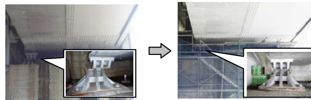
11.【橋桁のずれ(仙台駅構内)】
