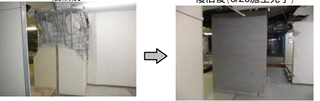
13.【高架橋柱の損傷(郡山駅事務所内)】
