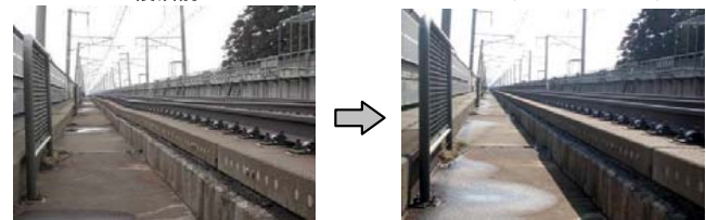
6.【軌道の変位(北上～新花巻間)】
