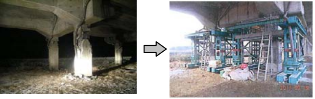
4.【高架橋柱の損傷(新花巻～盛岡間)】
