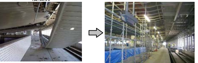
10.【天井材の落下(仙台駅ホーム)】
